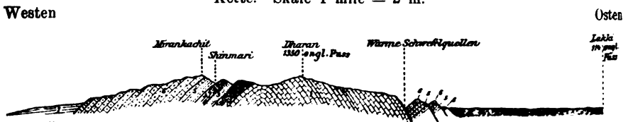
Fig. 1. Querprofil durch die Dharan-Antiklinale am Nordende der Lakki-Kette. Skale 1 mile = 2 m.
